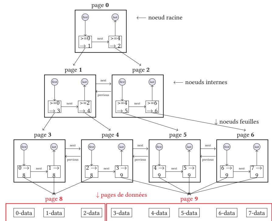
FIGURE 20 – Exemple de B^+
