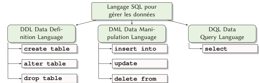
FIGURE 3 – Les ordres DDL, DML et DQL
