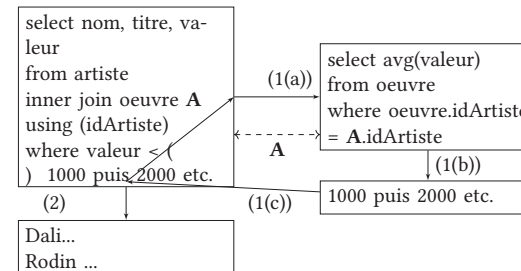
FIGURE 6 – Sous-requête corrélée
