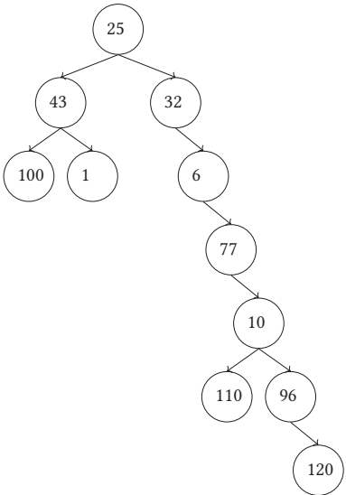
FIGURE 10 – Arbre binaire
