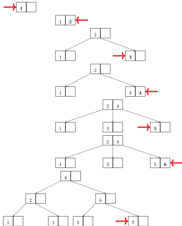
FIGURE 19 – Évolution du B-arbre après chaque insertion de clé
