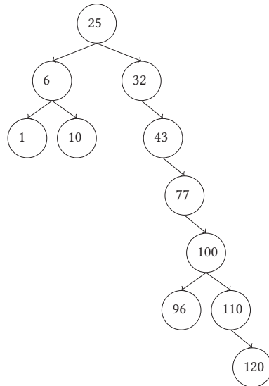
FIGURE 12 – Arbre binaire de recherche
