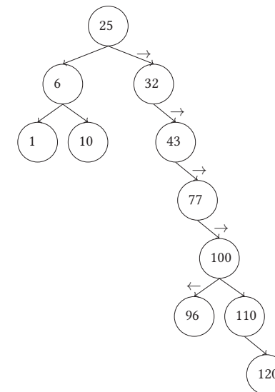
FIGURE 13 – Parcours d'un arbre binaire de recherche (clé 96)
