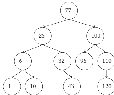
FIGURE 14 – Arbre binaire de recherche équilibré
