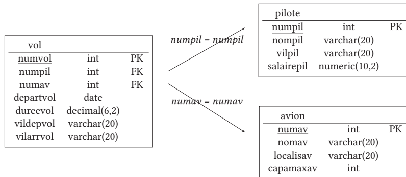
FIGURE 2 – Modèle Physique de la base de données des vols
