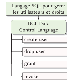
FIGURE 22 – Ordres SQL associés aux utilisateurs et privilèges
