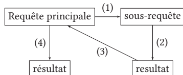
FIGURE 4 – Requête principale et sous-requête
