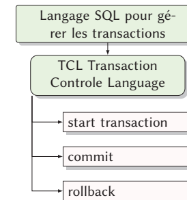
FIGURE 21 – Ordres SQL associés aux transaction
